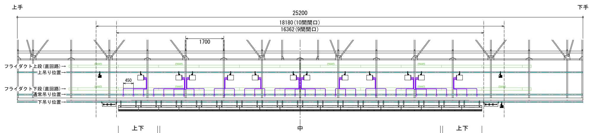
LB1 背面図 (積載荷重:1000kg) 縮尺: 1:100
