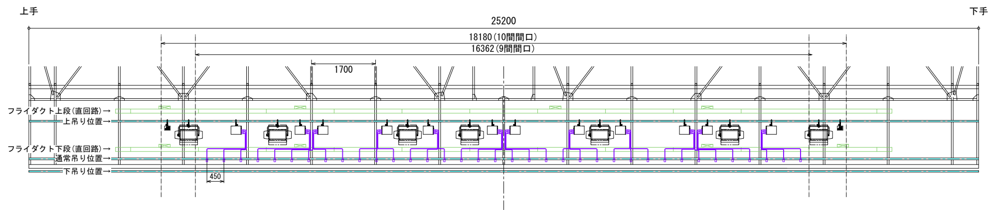
LB3 背面図 (積載荷重:1000kg) 縮尺: 1:100
