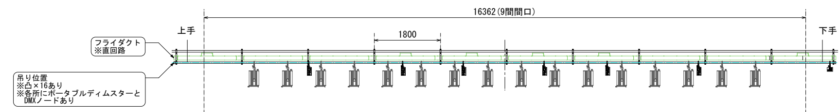
PS 背面図 (積載荷重:400kg) 縮尺: 1:100
