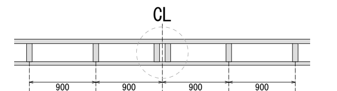
美術ボタンCL部分 正面図 (ボタン3, 6, 16以外のボタン) 縮尺: 1:50 (積載荷重:500kg)
