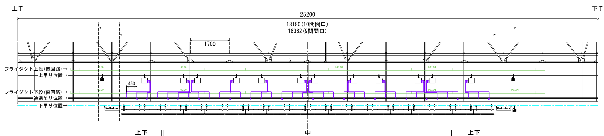
LB2 背面図 (積載荷重:1000kg) 縮尺: 1:100
