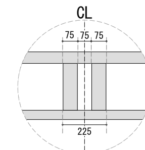
美術ボタンCL部分 拡大図 縮尺: 1:20
