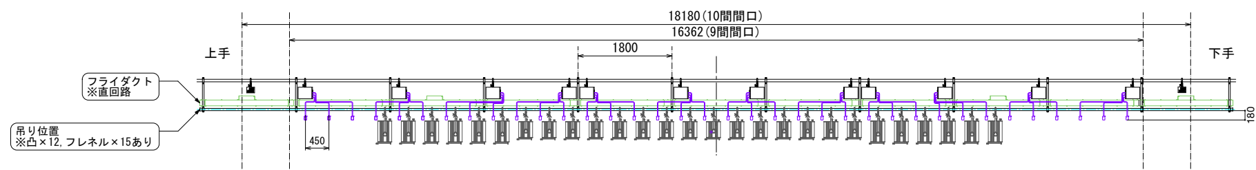
4SUS 背面図 (積載荷重:380kg) 縮尺: 1:100
